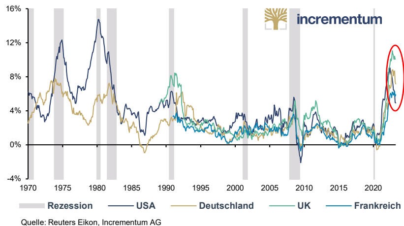
CPI/VPI, yoy, USA, Deutschland, UK, Frankreich, 01/1970-04/2023
